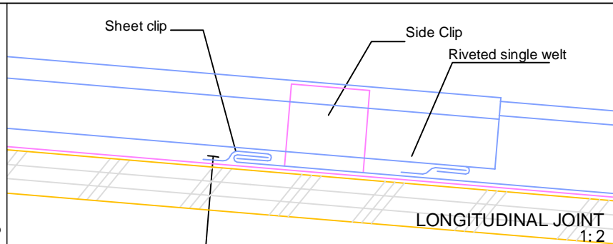
CLIP
